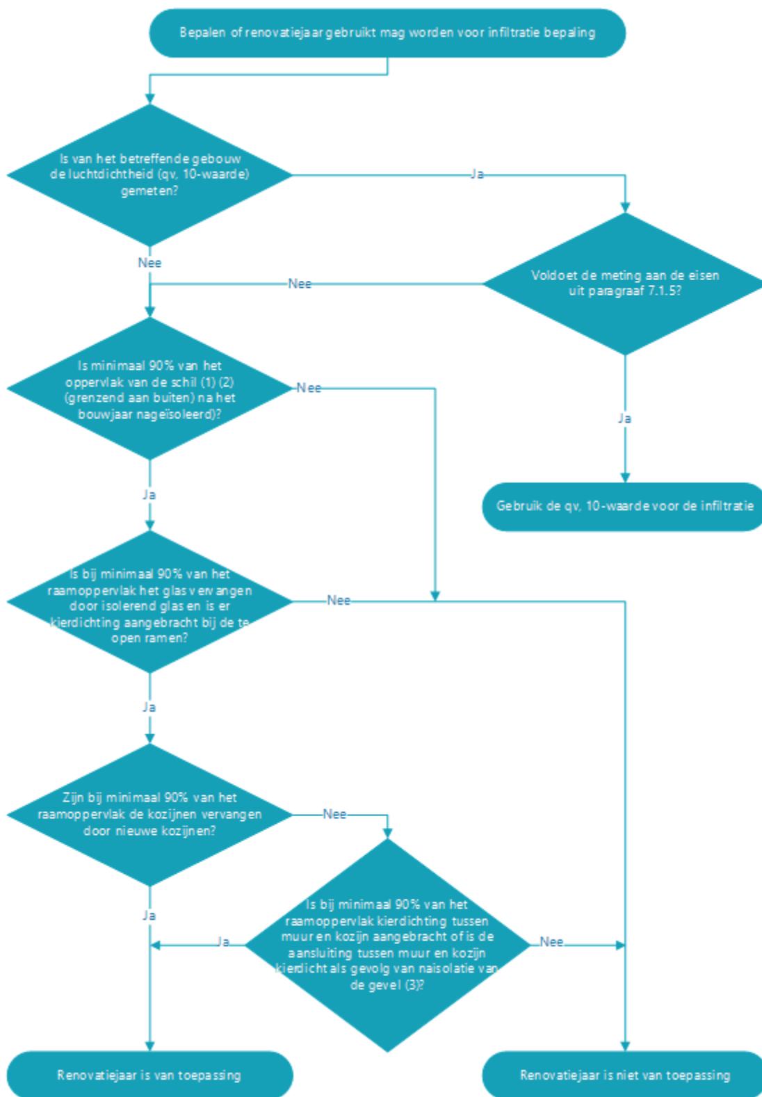
Afb. 7.2 Beslisschema voor het gebruik van renovatiejaar bij bepaling infiltratie
