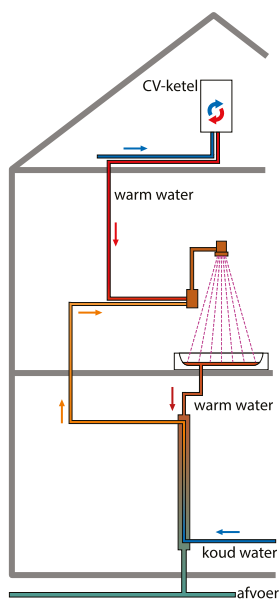
Afb. 13.2 DWTW-unit aangesloten op alleen koudepoort douchemengkraan
