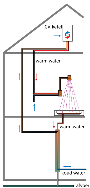
Afb. 13.3 DWTW-unit aangesloten op alleen inlaat van het toestel
