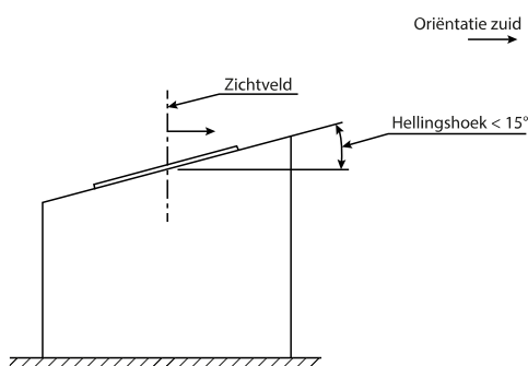
Afb. 16.2 Bijzondere situatie 1, met hellingshoek < 15°
