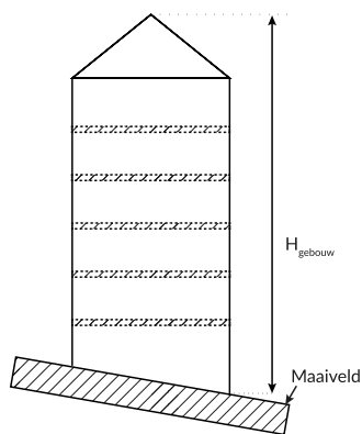
Afb. 7.3 Bepalen van de gebouwhoogte bij ongelijk maaiveld
