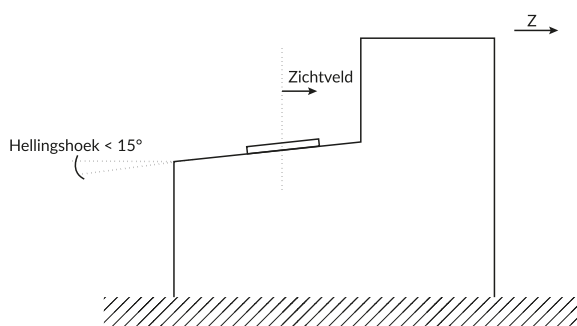
Afb. 16.3 Bijzondere situatie 2, met hellingshoek < 15°
