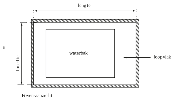
Afb. 7.7 Gebruiksoppervlakte zwembad, bovenaanzicht
