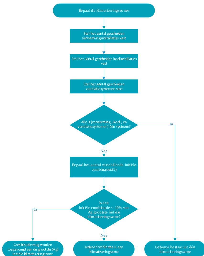
Afb. 6.5 Beslisschema voor de bepaling van klimatiseringszones
