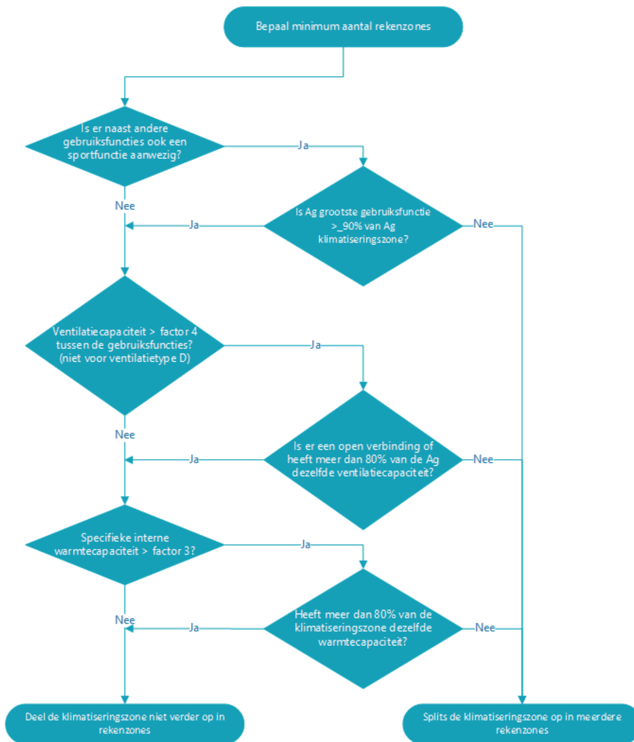
Afb. 6.6 Beslisschema voor het minimum aantal te hanteren rekenzones
