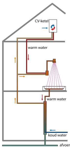
Afb. 13.1 DWTW-unit aangesloten op zowel koudepoort douchemengkraan als inlaat van het toestel
