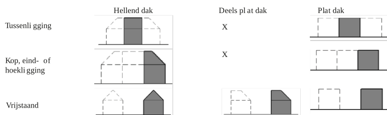
Afb. 7.1 Te bepalen gegevens dakconstructies bij enkellaags utiliteitsgebouwen
