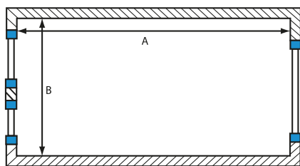
Afb. 7.6 Meten tussen de opgaande scheidingsconstructies
