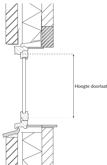
Afb. 11.2 Bruto hoogte van de doorlaat (verticale doorsnede opening)
